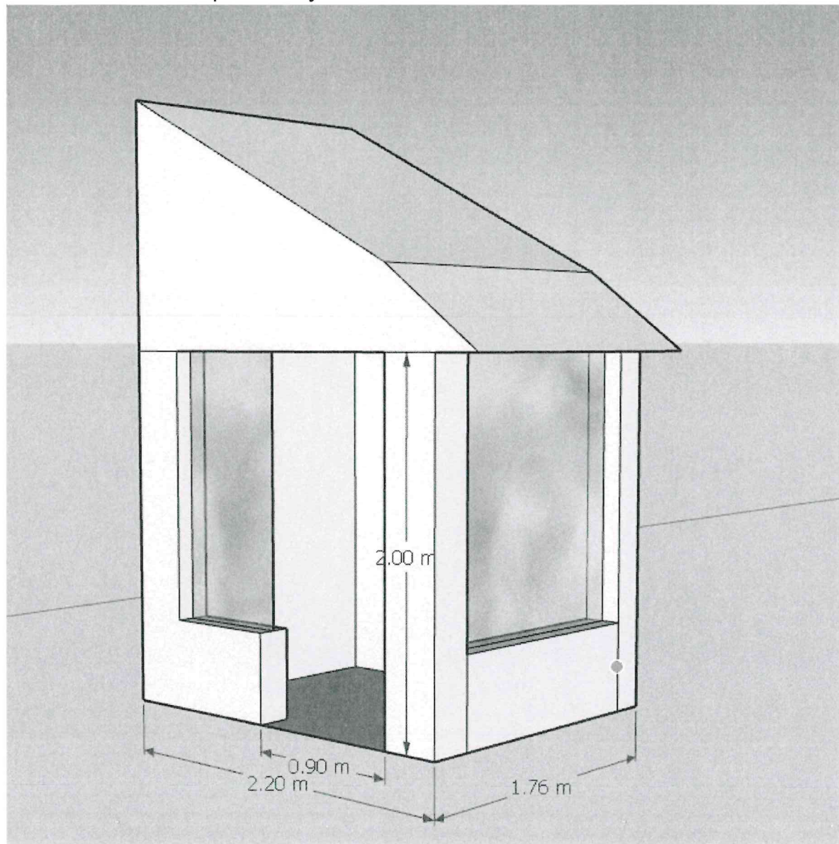
imagen 1 modelo de infraestructura y medidas de puertas
